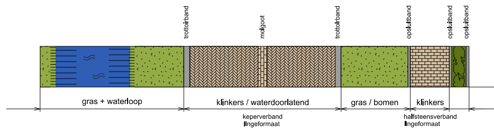
PROFIEL B-B
