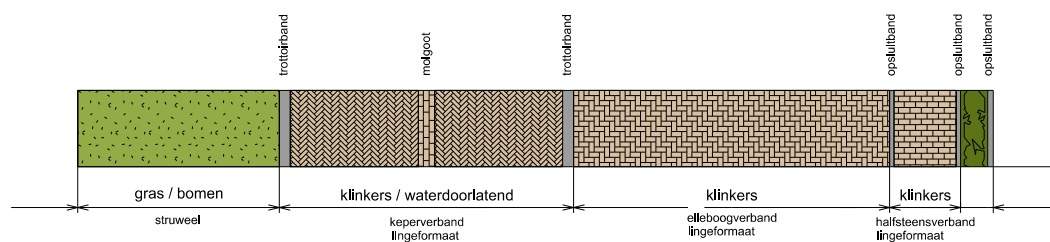
PROFIEL A-A
