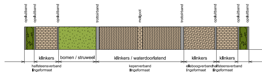
PROFIEL B
