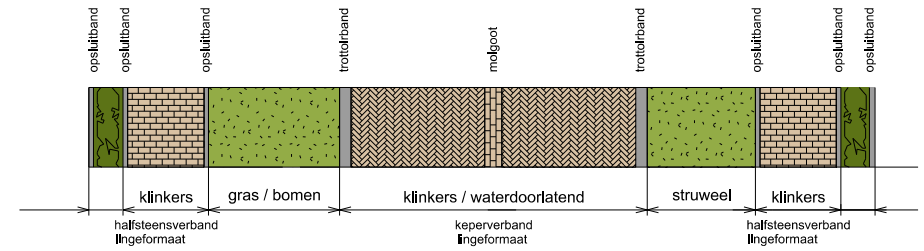
PROFIEL C
